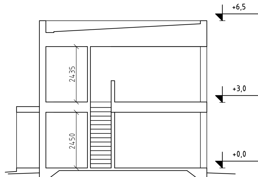
principsektion
