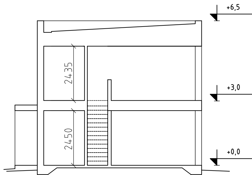
principsektion
