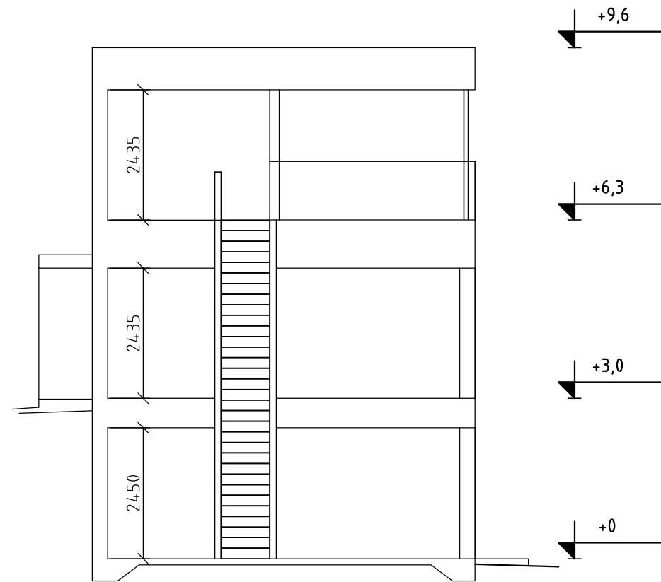
principsektion
