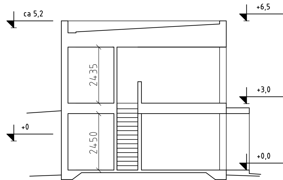
principsektion
