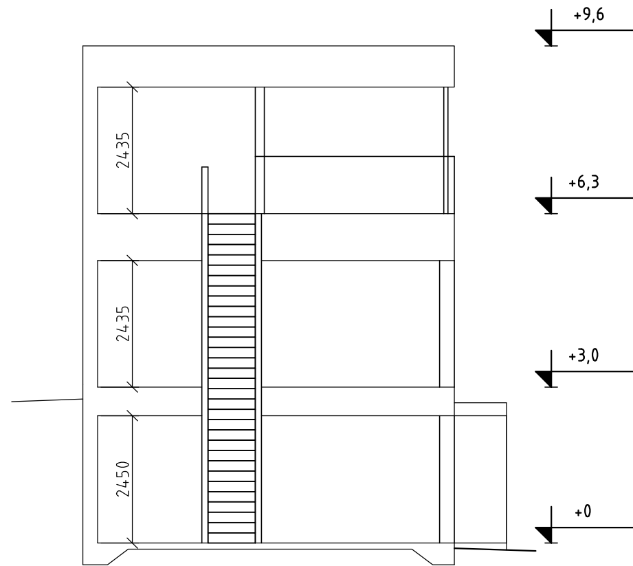
principsektion
