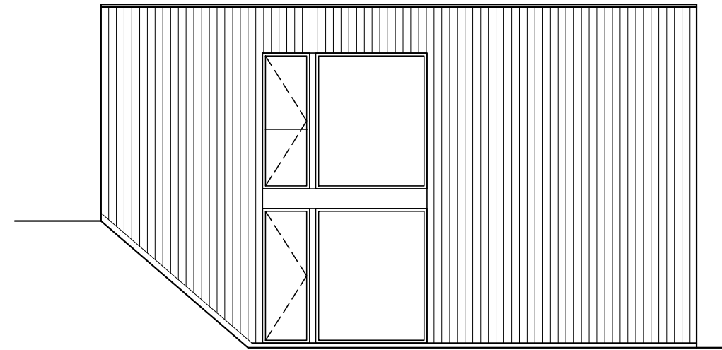
fasad B
