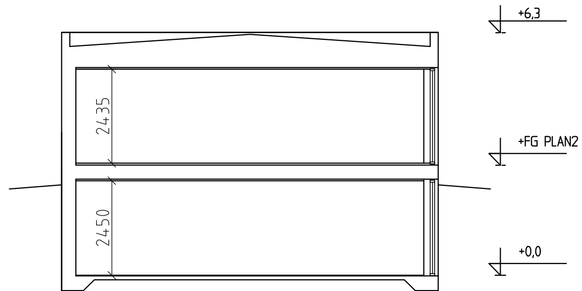
principsektion B-B
