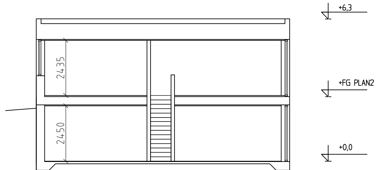
principsektion A-A
