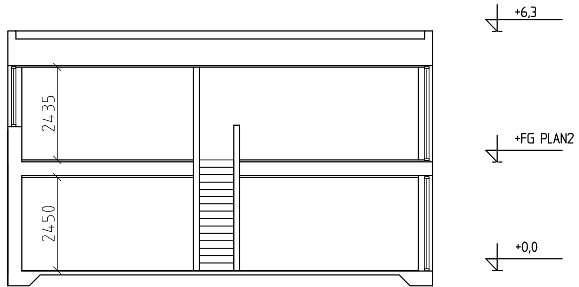
principsektion A-A
