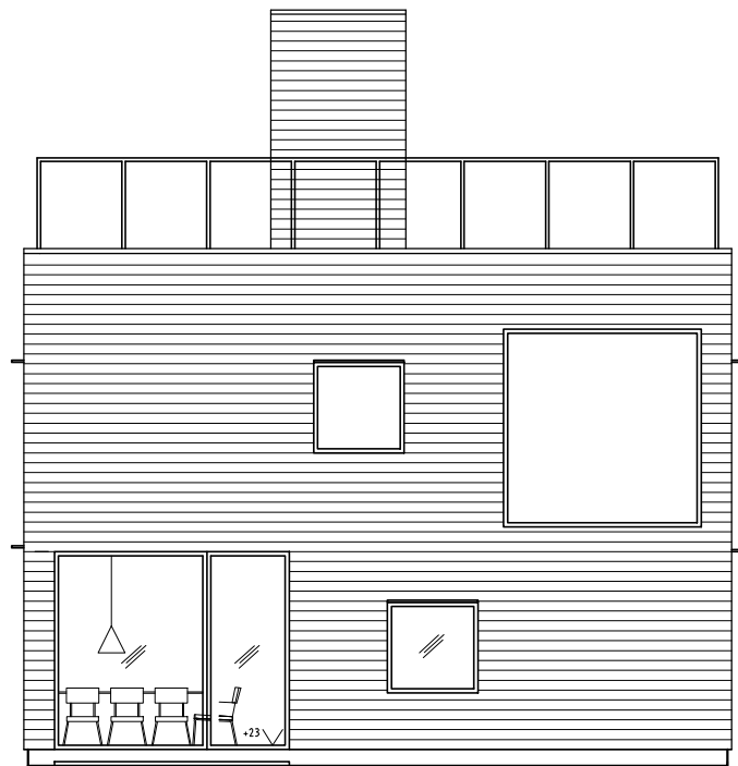
fasad C
