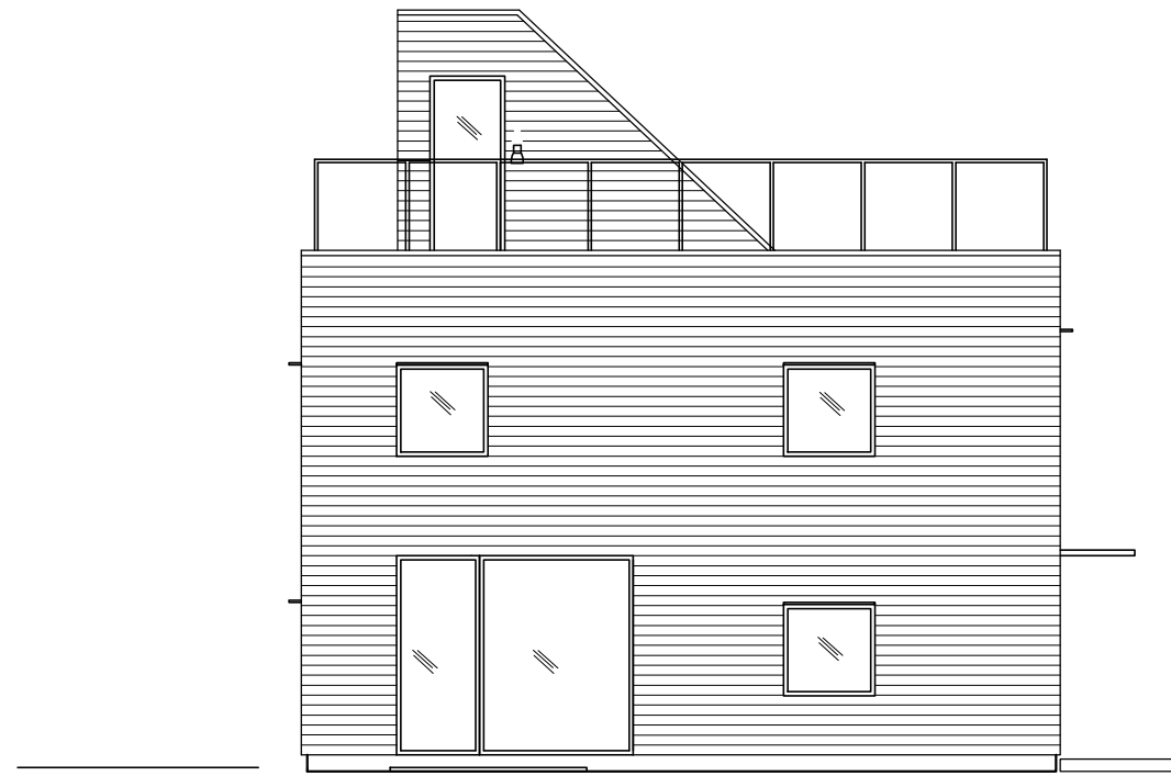
fasad B
