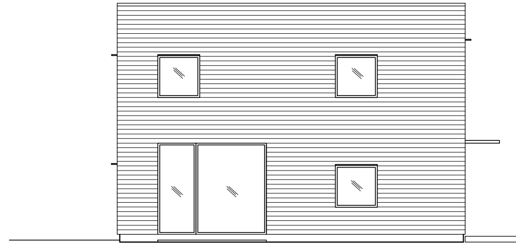
fasad B
