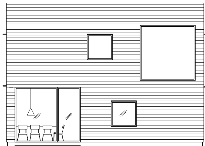
fasad C
