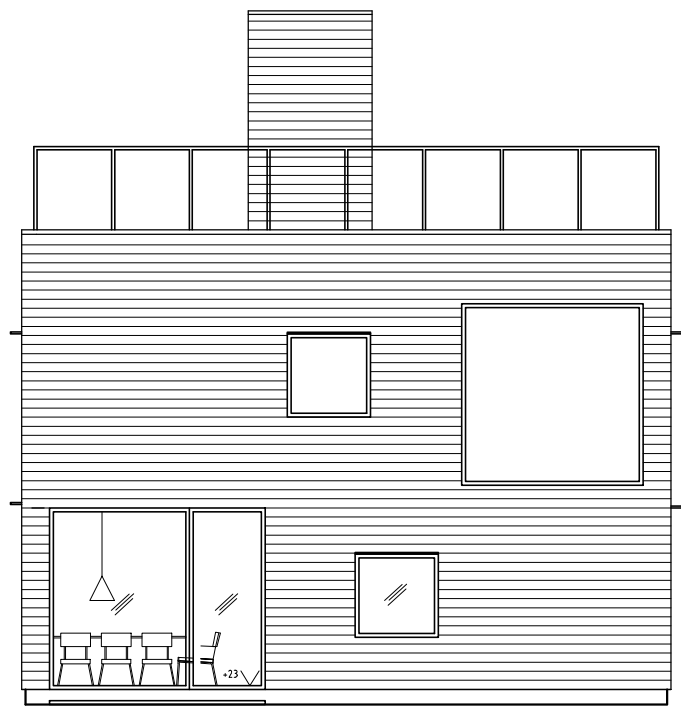
fasad C
