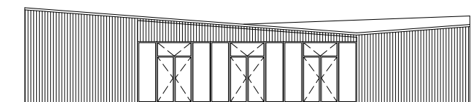
fasad C
