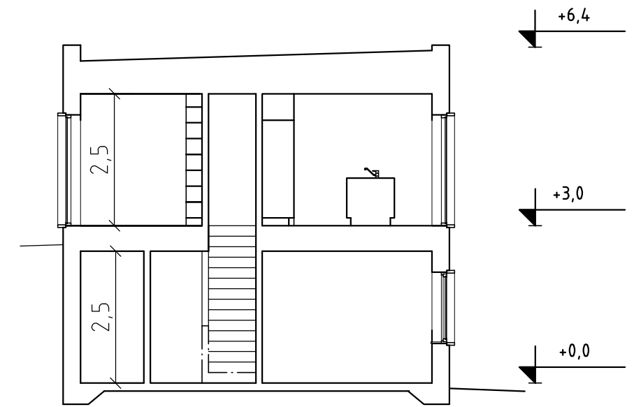
sektion B-B
