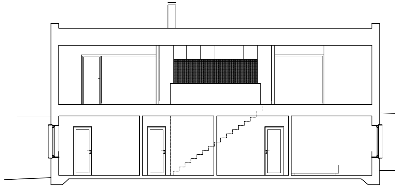
sektion A-A
