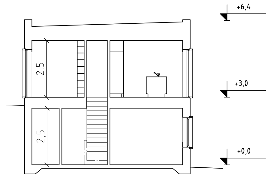
sektion B-B
