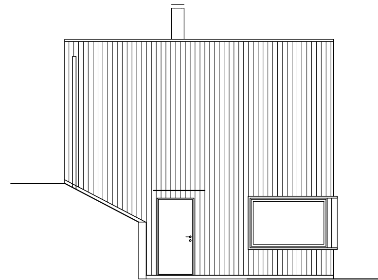
fasad B
