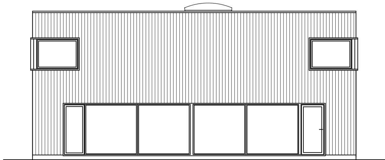
FASAD C
