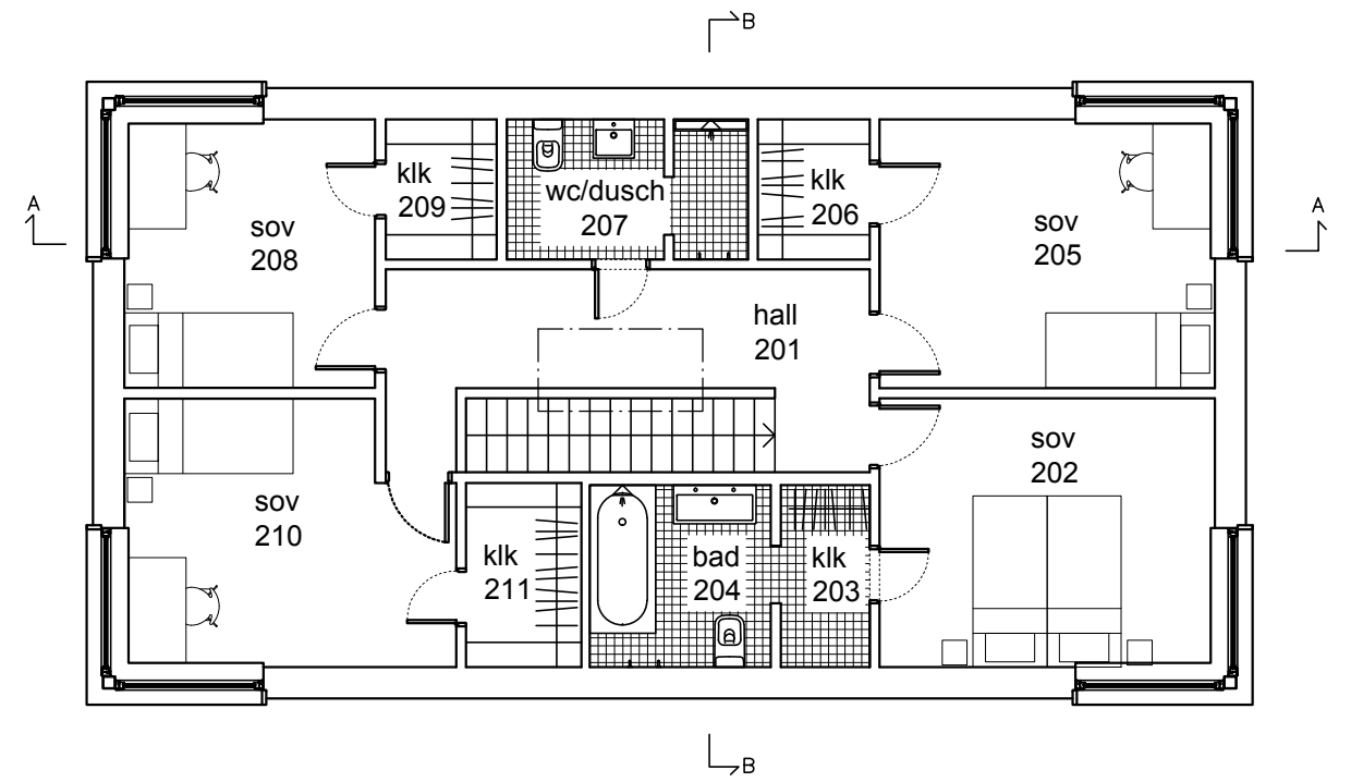
övre plan
