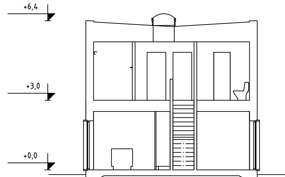
sektion B-B
