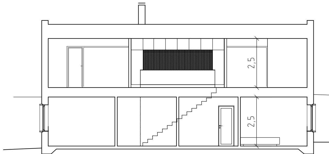
sektion A-A
