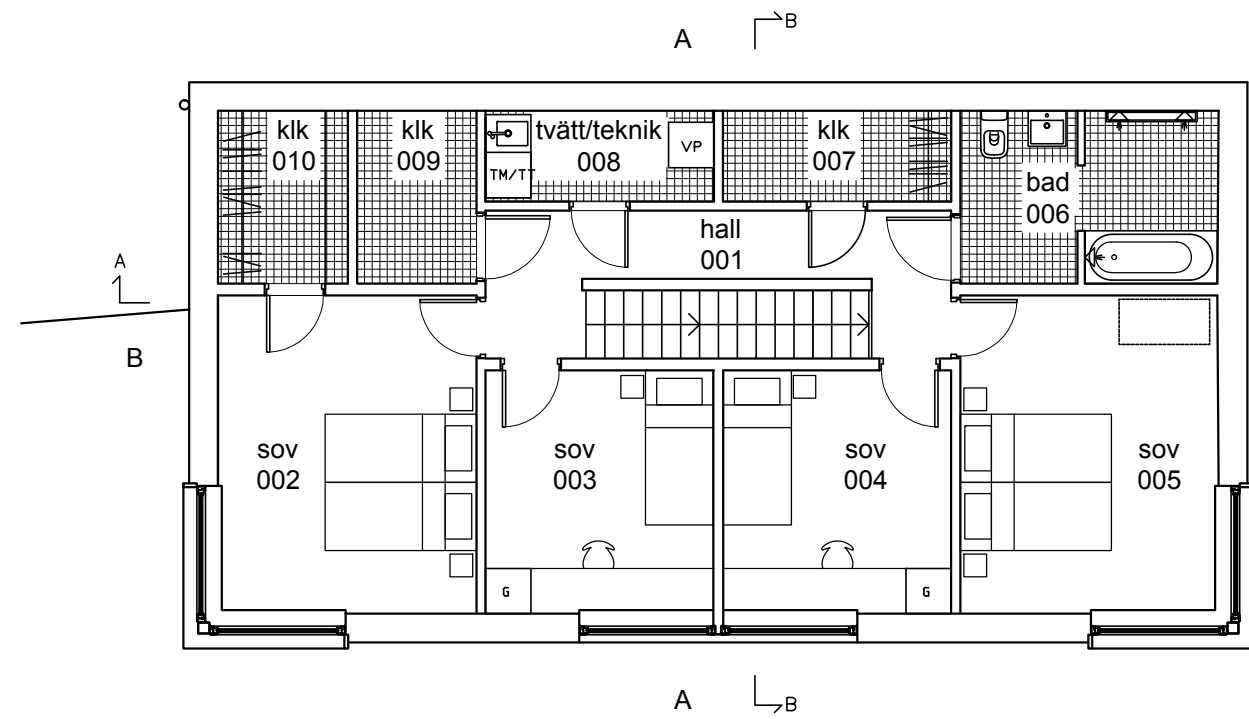
souterrängplan
