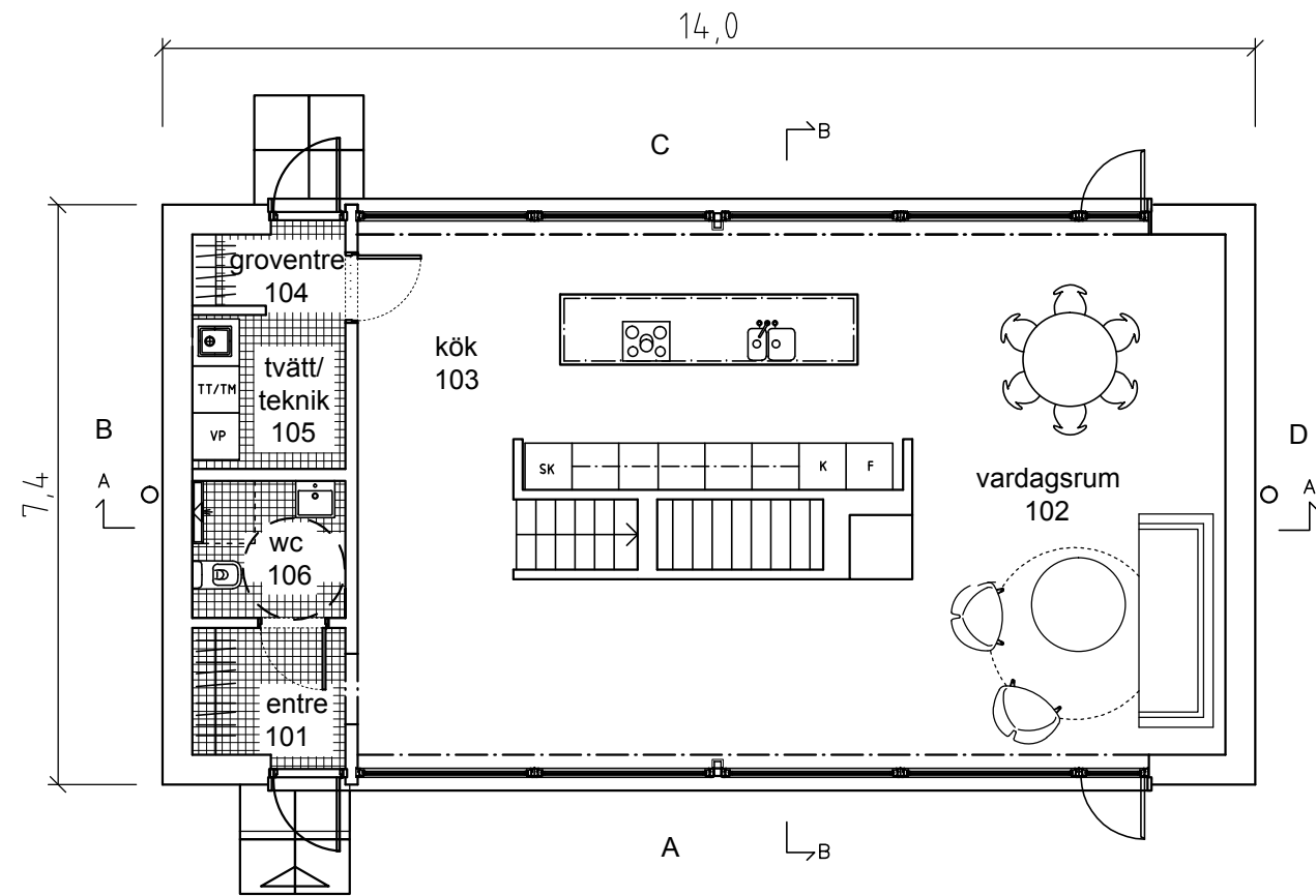
entréplan
