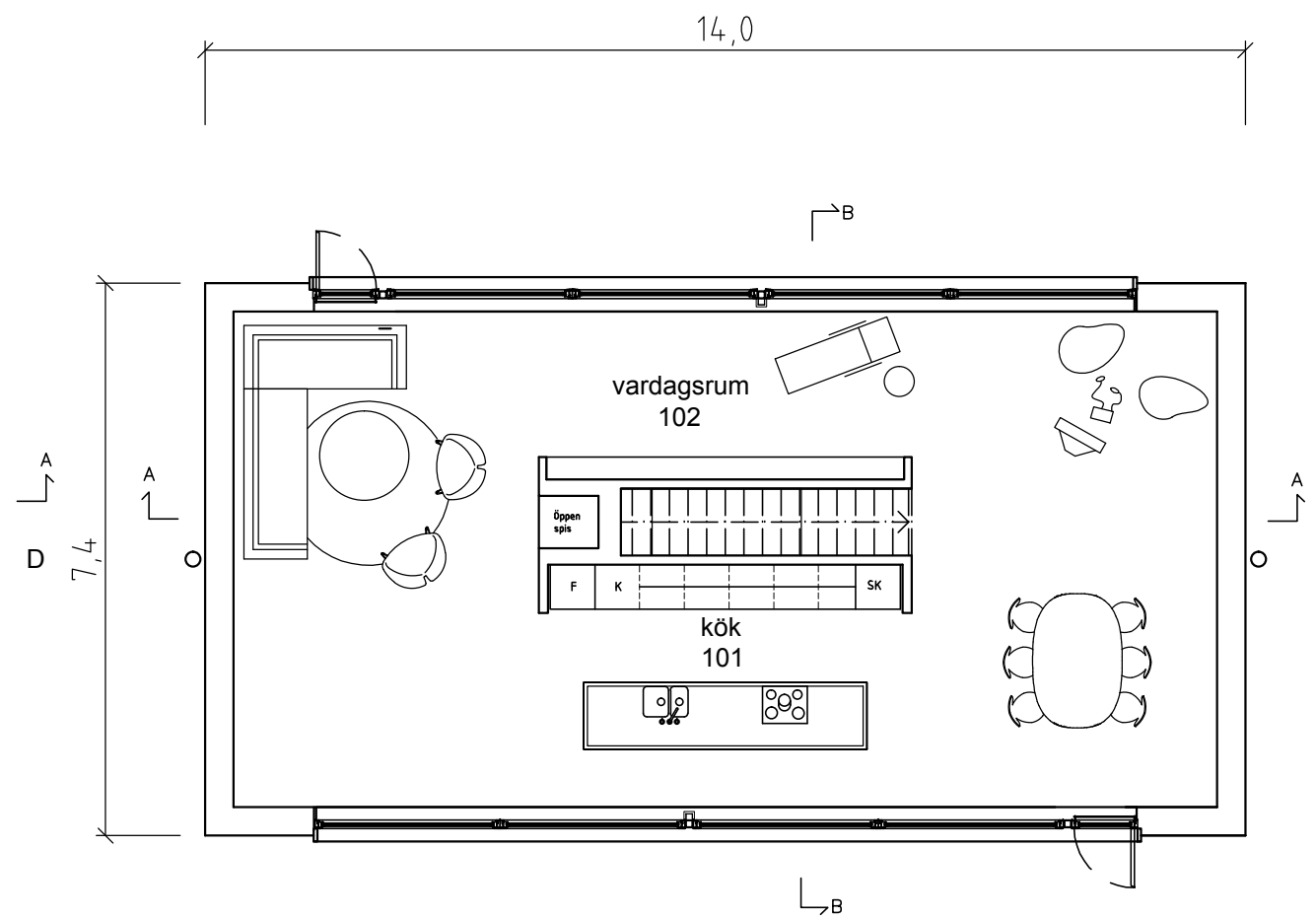
övreplan
