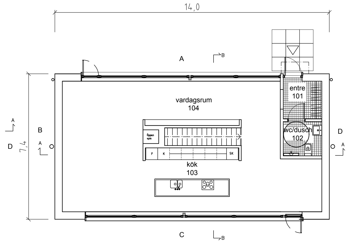
övreplan
