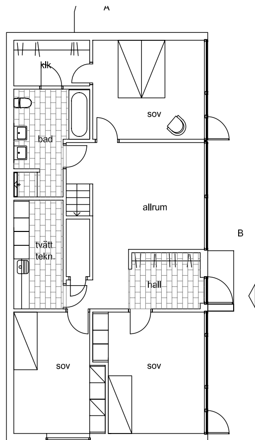
sueterängplan
