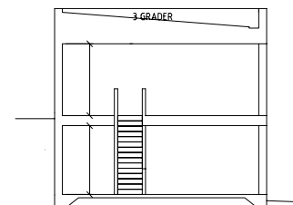
prindelsektion
