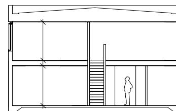
principsktion
