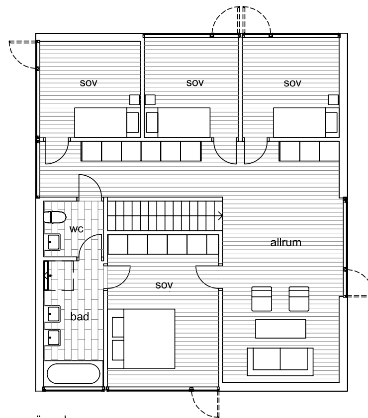
övreplan
