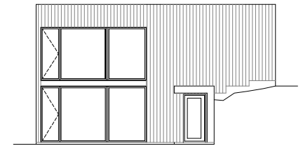
fasad D
