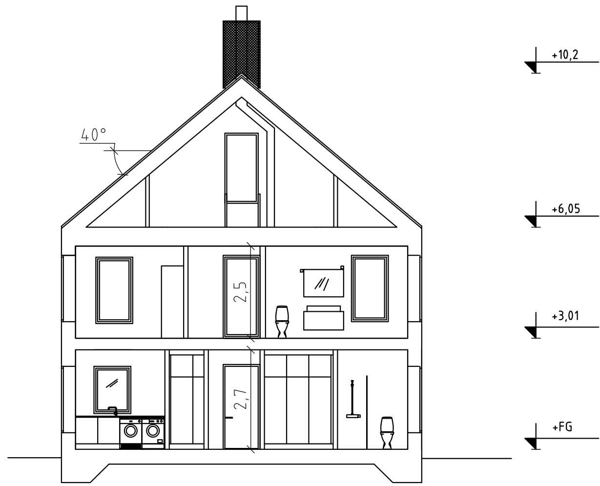
principsektion
