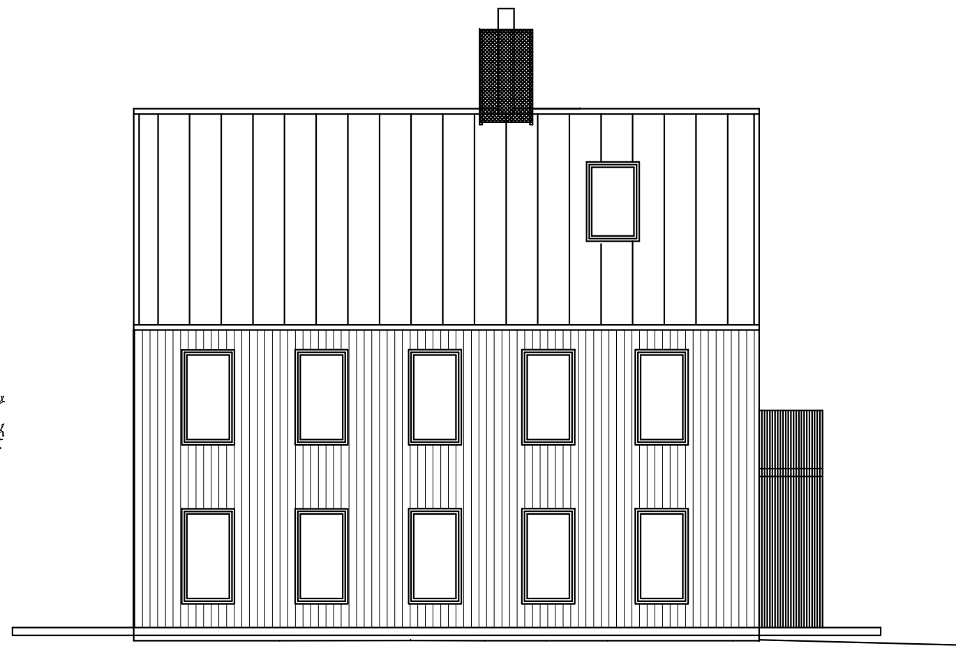
fasad B
