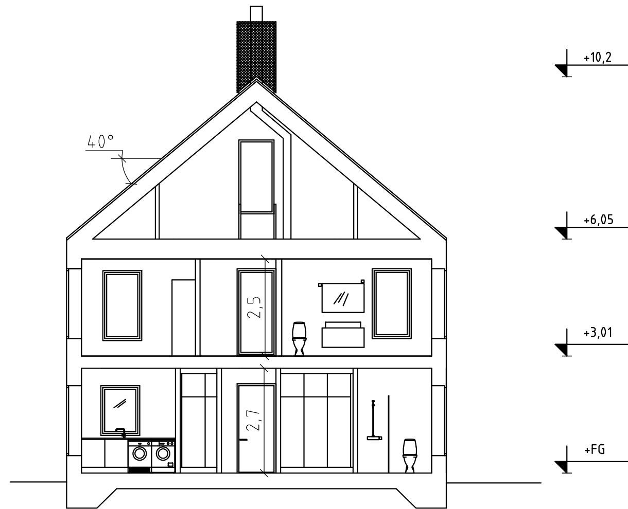
principsektion
