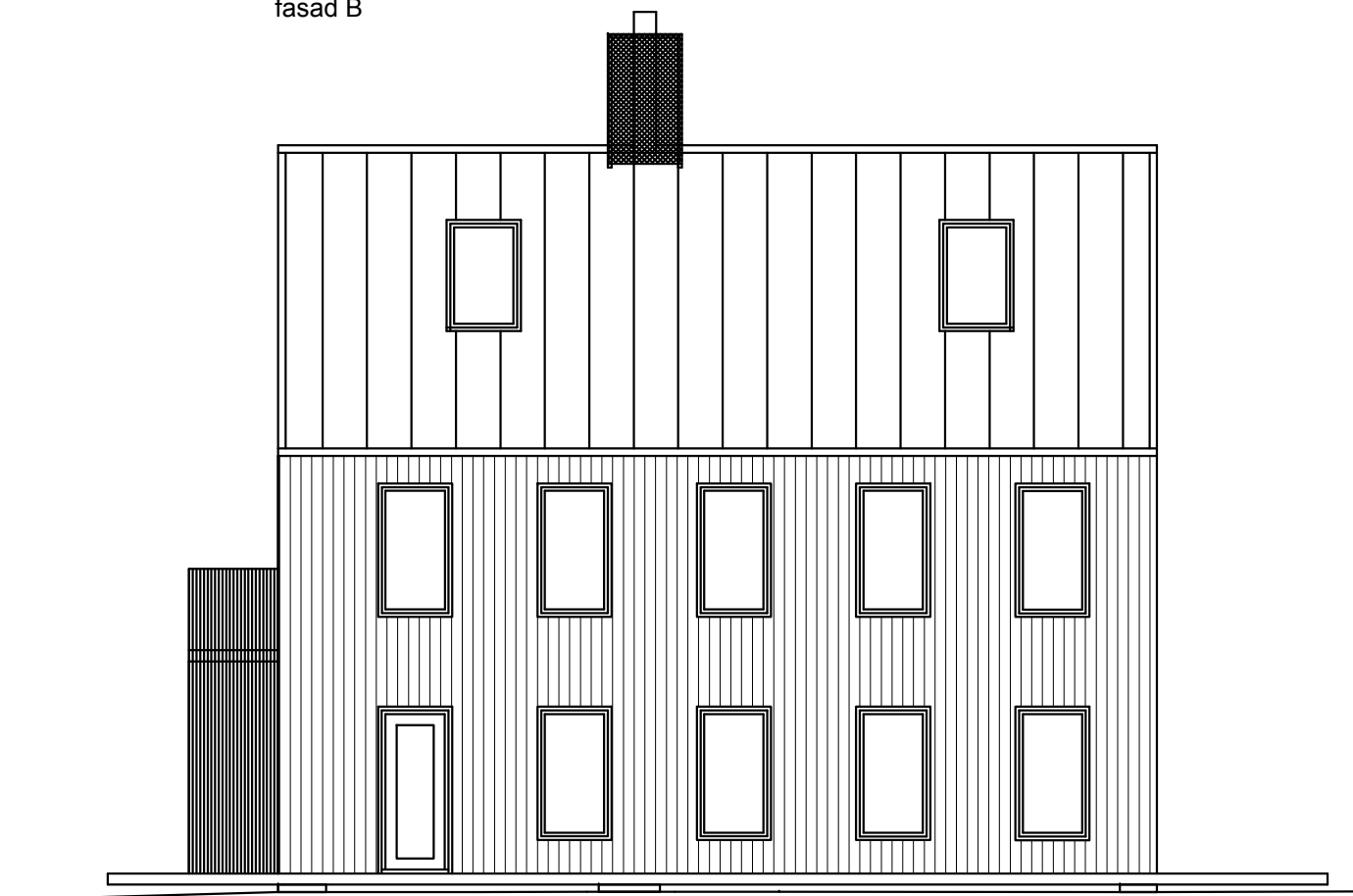
fasad B
