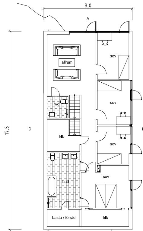
suterrängplan
