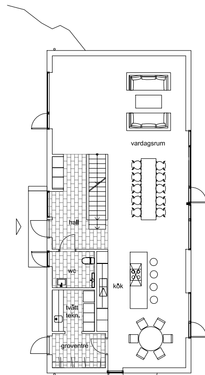
övre plan
