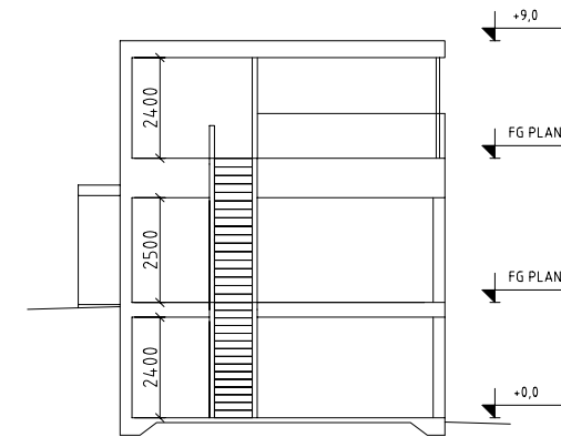
principsektion
