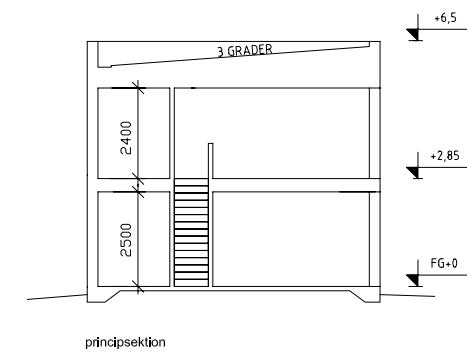
princpsektion
