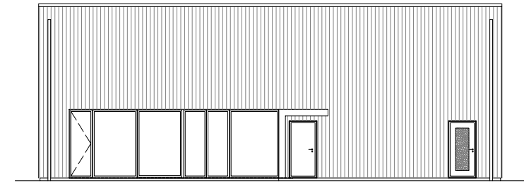
fasad D
