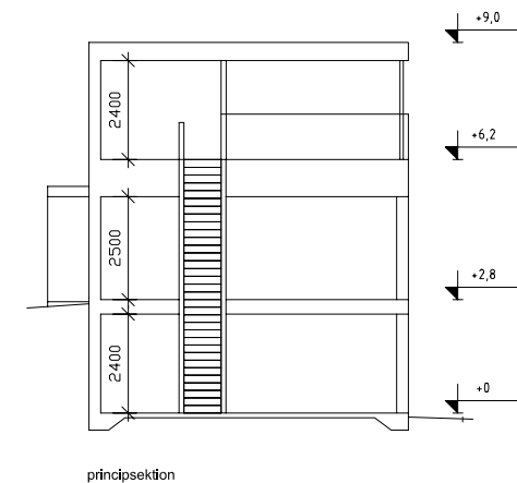
principsektion
