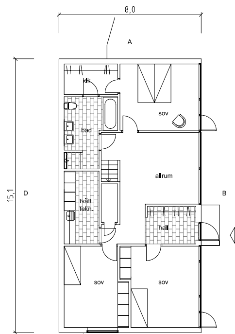
suterängplan
