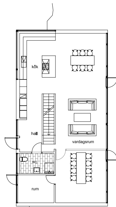
övre plan
