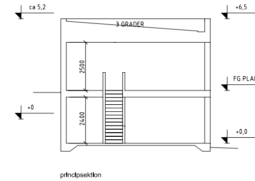
principsnitt
