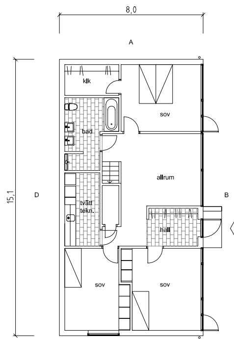
suterrängplan
