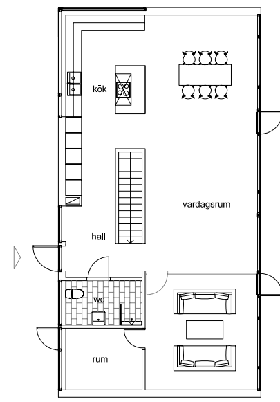
övre plan
