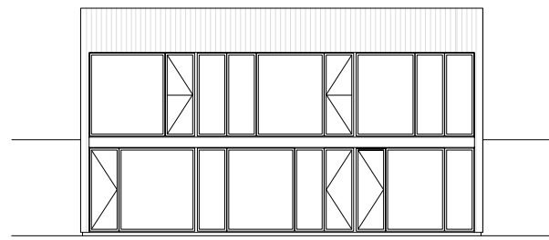
fasad B
