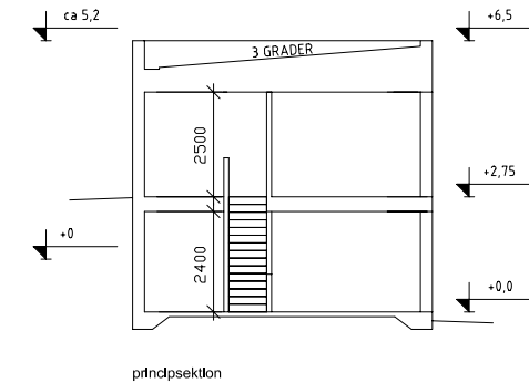
principsnitt
