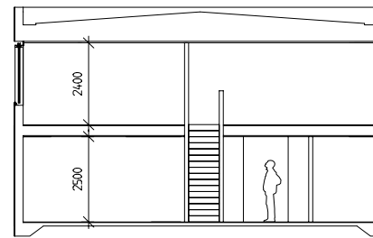
principsektion
