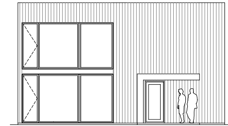
fasad D
