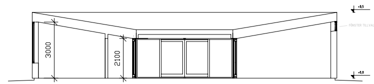
principsektion
