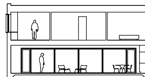
sektion A-A
