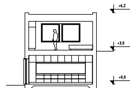
sektion B-B
