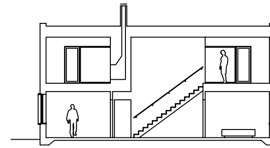
sektion A-A
