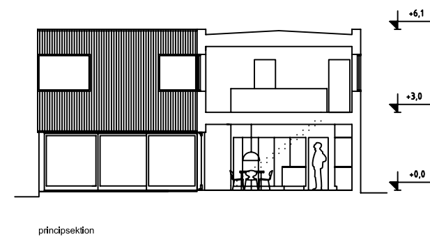
principsektion
