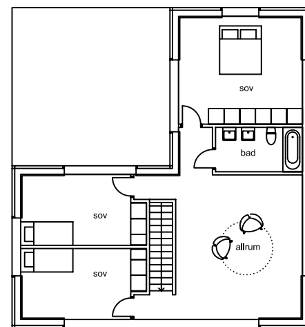
övreplan
