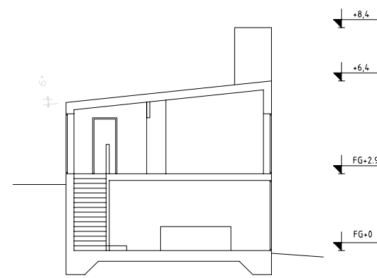
principsktion
