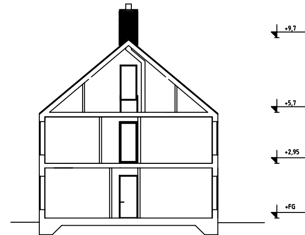
principsktion
