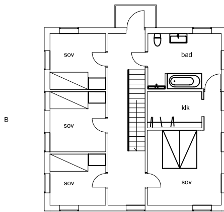
övreplan
