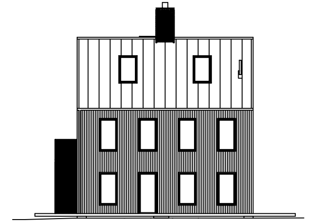
fasad D
