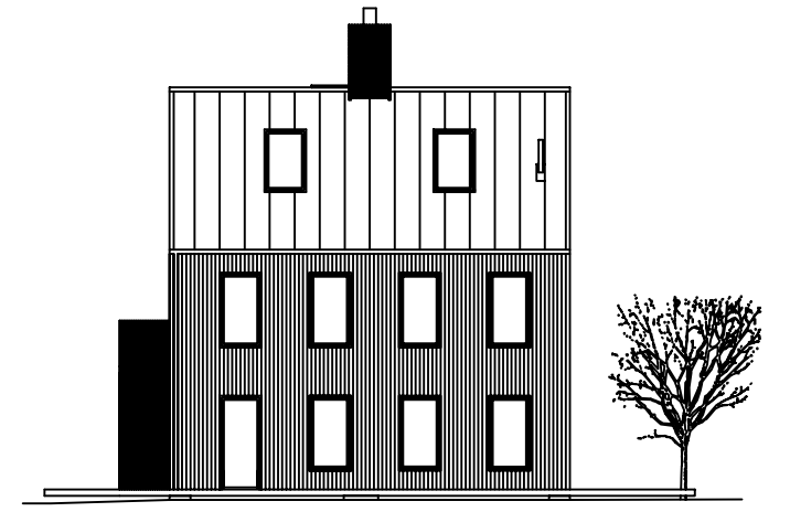
fasad D
