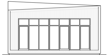
fasad D
